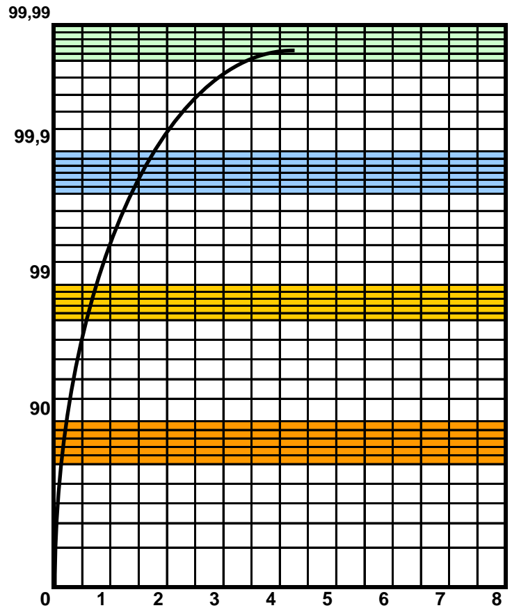
Curva eficiencia (%)
